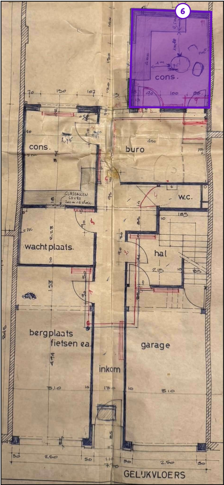
Legende van plan 1.4: Plafond plaat - gelijkvloers
