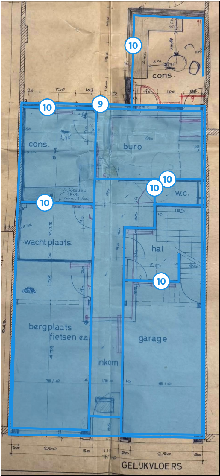
Legende van plan 1.3: Bezetting muur - plafond gelijkvloers
